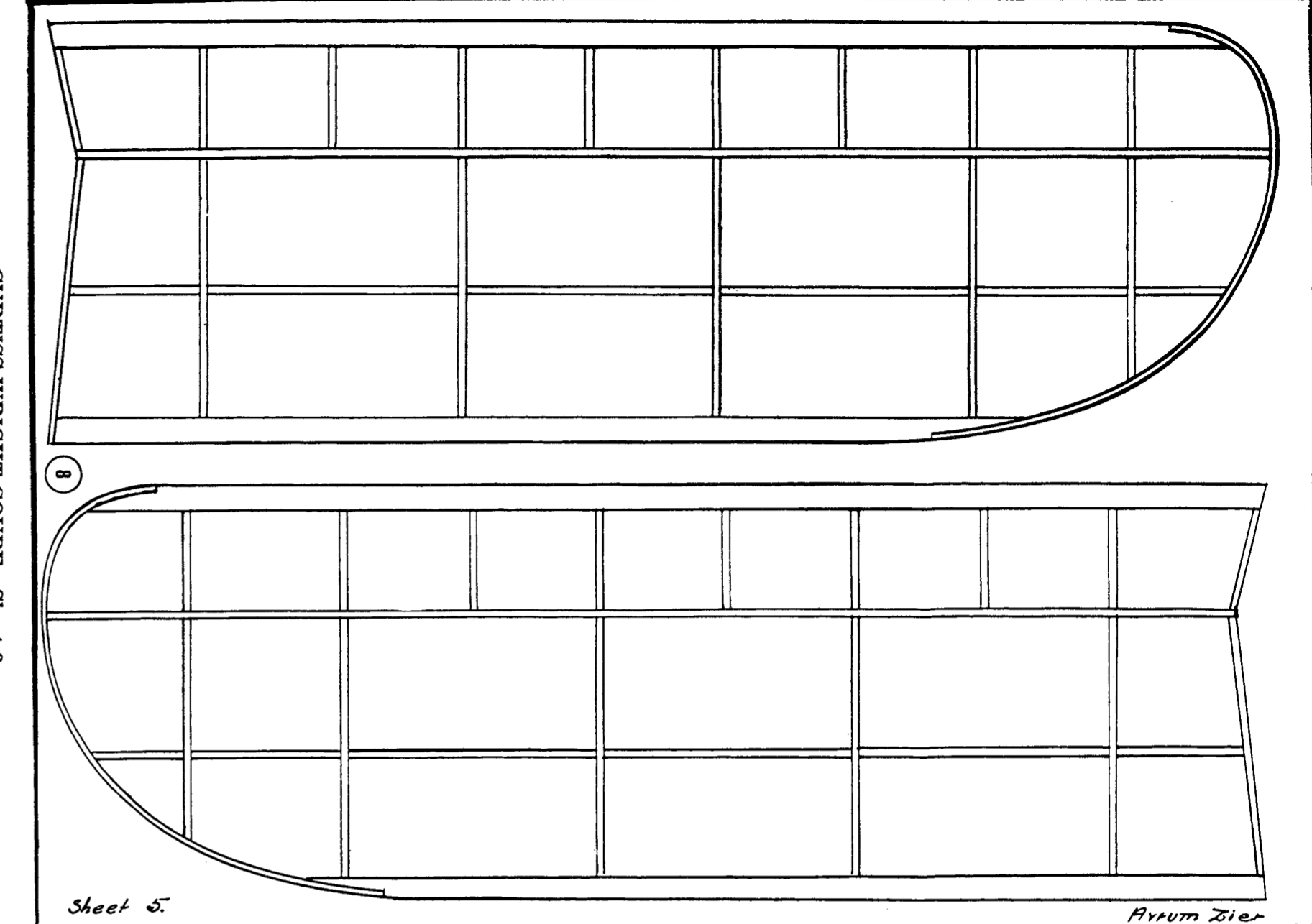
CURTISS-WRIGHT COUPE—Sheet 5
