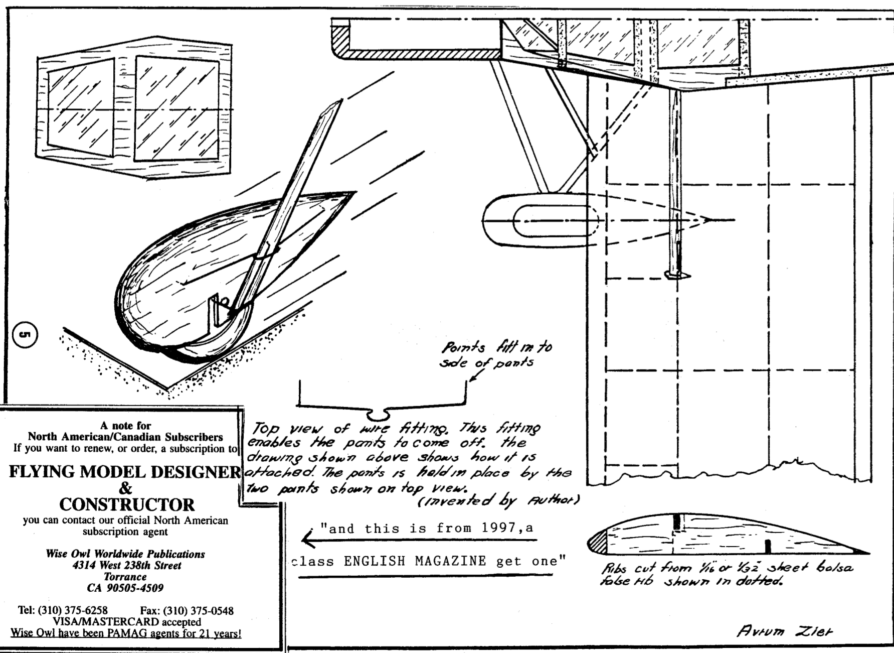
CURTISS-WRIGHT COUPE—Sheet 2
